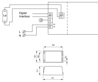
Technische Daten Philips HID-DV PROG Xt 250 SON C2 208-277V für 250W
